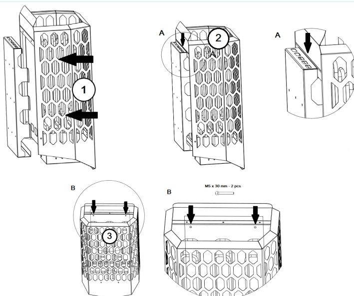
Abb. 3 Montage des Ofens in einer Wandhalterung.
