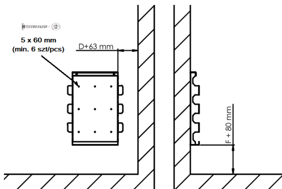
Rys. 2 Rozmieszczenie otworów pod uchwyt ścienny pieca.
