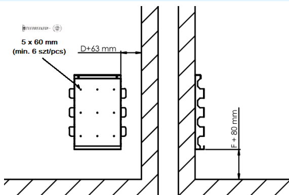
Abb. 2 Position der Bohrungen für die Wandhalterung des Ofens.
