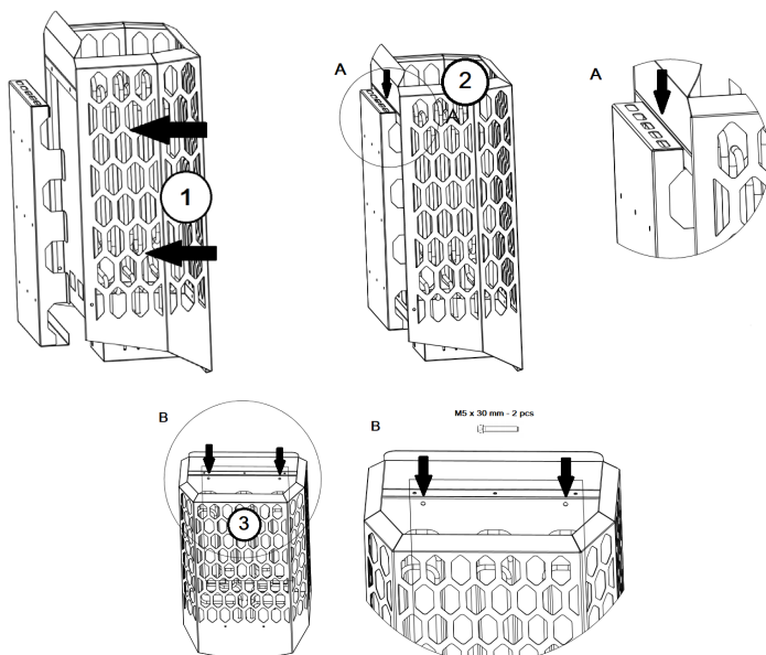
Rys. 3 Montaż pieca w uchwycie ściennym.
